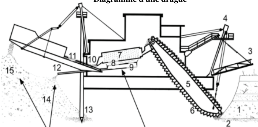
Diagramme d'une drague
